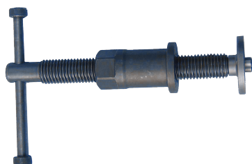
01435L-1 Jobbraforgató orsó
